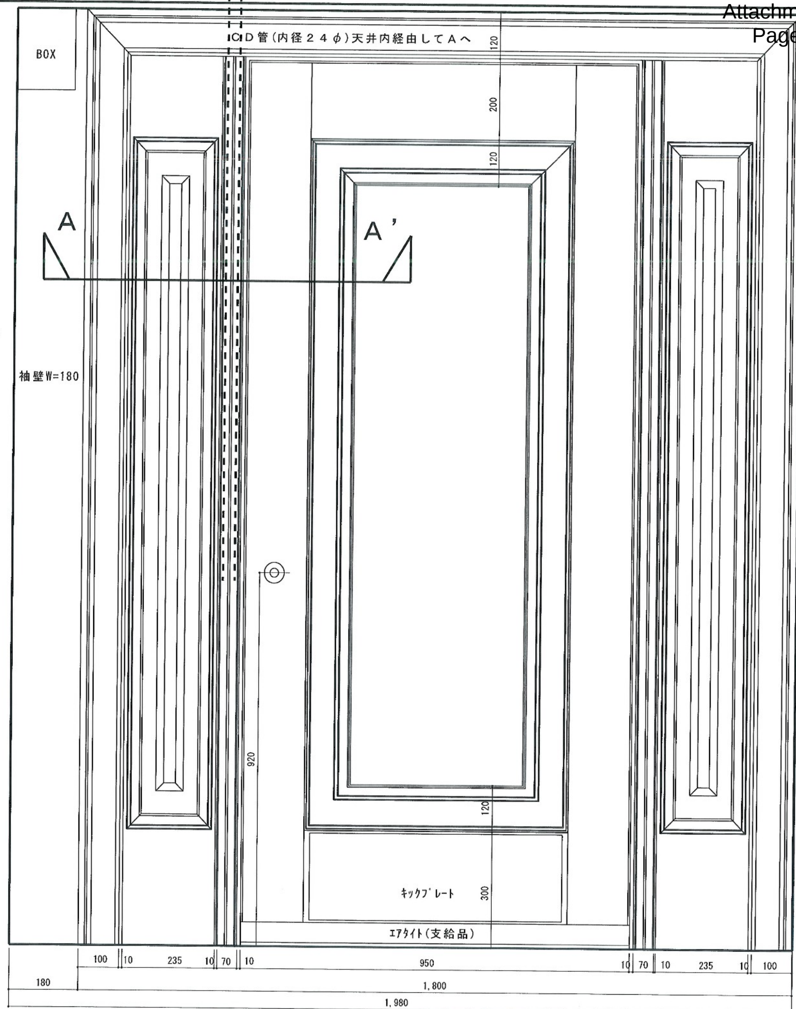
エントランスドア姿図 S = 1 / 10
